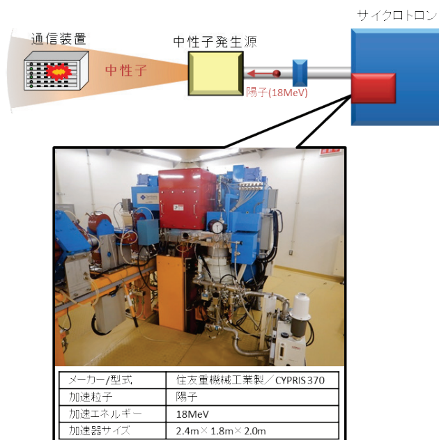
図 2 SHIEI 所有の小型加速器中性子源を用いたソフトエラー試験系
